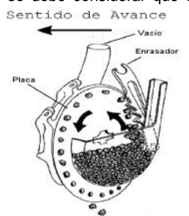
Fig. 1: Distribuidor neumático de succión, con placa de acero inoxidable y engrasador.
