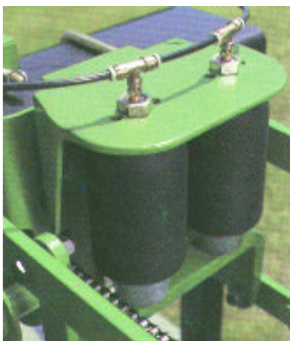
Figura 12: Pulmones neumáticos con carga constante en los paralelogramos de la sembradora de grano grueso. Tendencia en el desarrollo para mejorar la uniformidad de profundidad de implantación.
